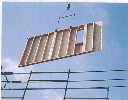
▲パネルの吊り上げ
