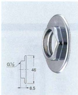
ネジフランジ(小)
